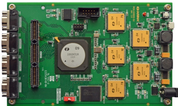
Отладочный модуль MCK-02REM-3U
