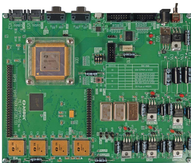
Отладочный модуль MCT-03PEM-6U
