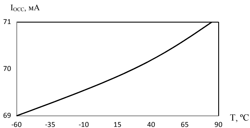
Рисунок 7.4. Зависимость динамического тока потребления от температуры при F_{RFD}=100 МГц, U_{CCD} = U_{CCA} = U_{CCK} = 3,47 В
