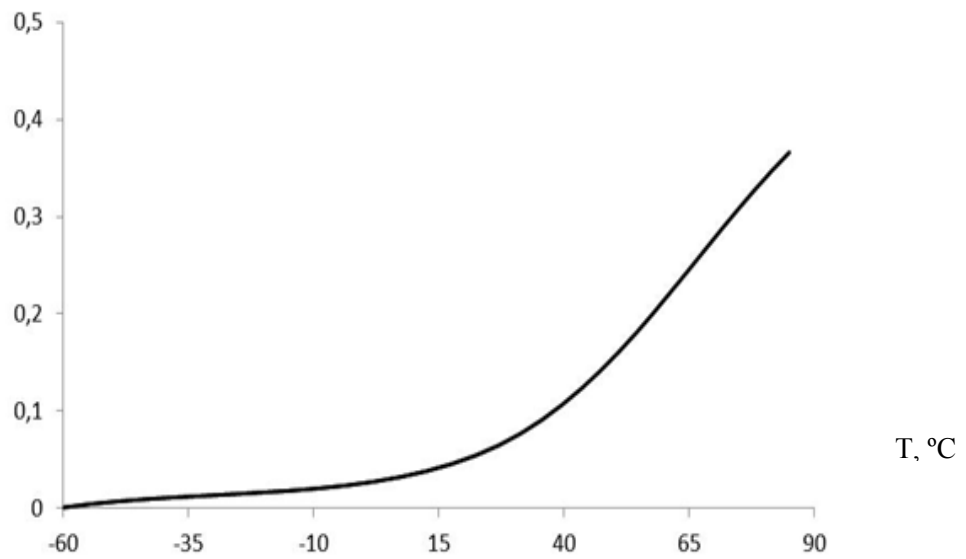
Рисунок 7.8. Зависимость тока утечки высокого уровня I_{IH} от температуры при U_{IH}=3,67 В, U_{CCD} = U_{CCA} = U_{CCK} = 3,47 В
