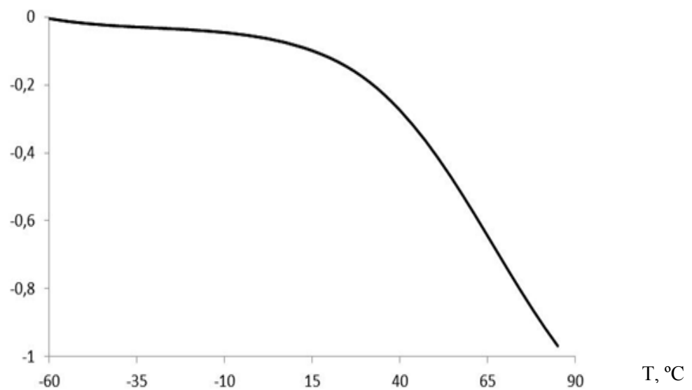
Рисунок 7.9. Зависимость тока утечки низкого уровня I_{IL} от температуры при U_{IL} = \text{минус } 0,2 В, U_{CCD} = U_{CCA} = U_{CCK} = 3,47 В
