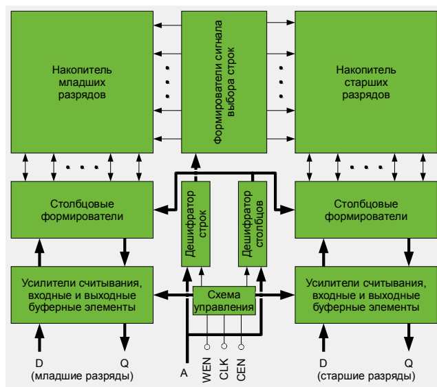
Общая структурная схема всех блоков однопортовой памяти
