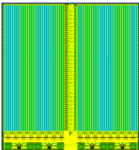
Топология СФ-блока с организацией 2Кх8
